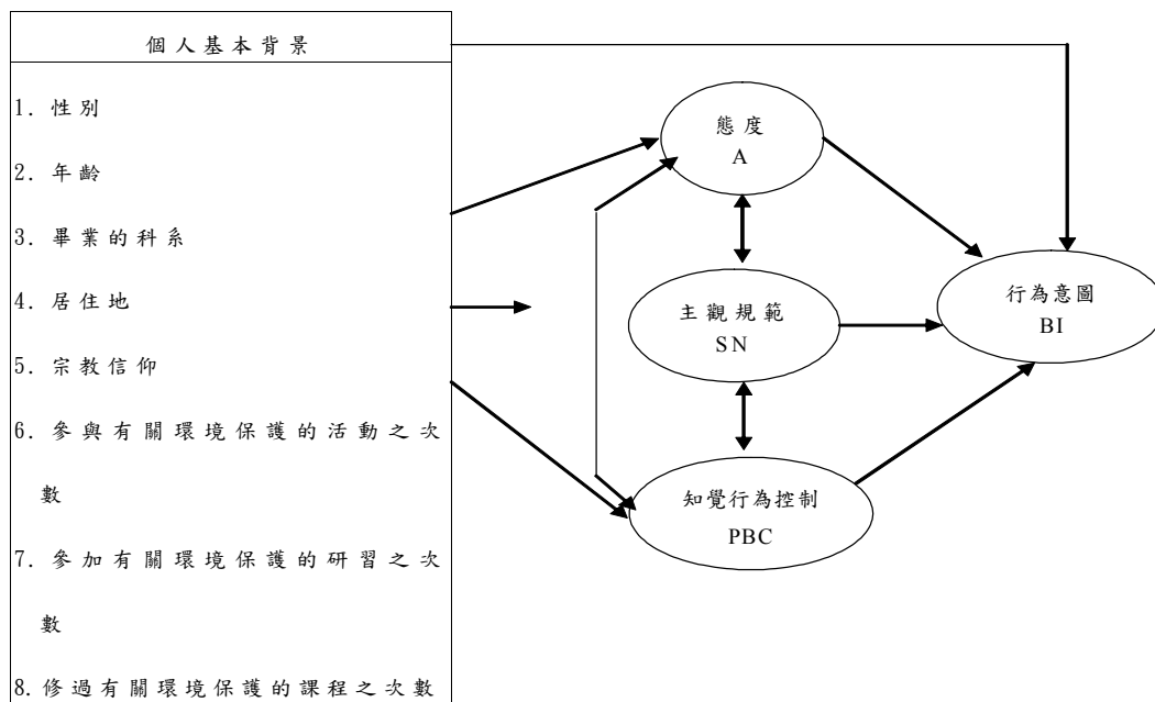
圖 1 研究架構圖
